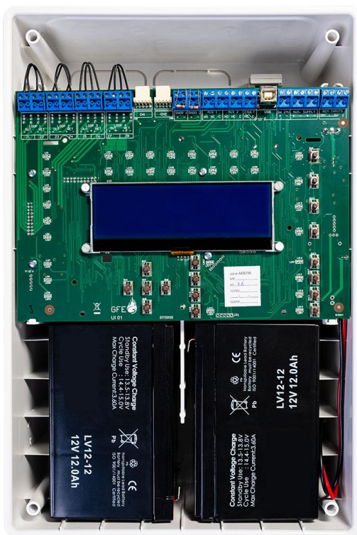
PLACA PRINCIPAL + BATERIAS INTERNAS
