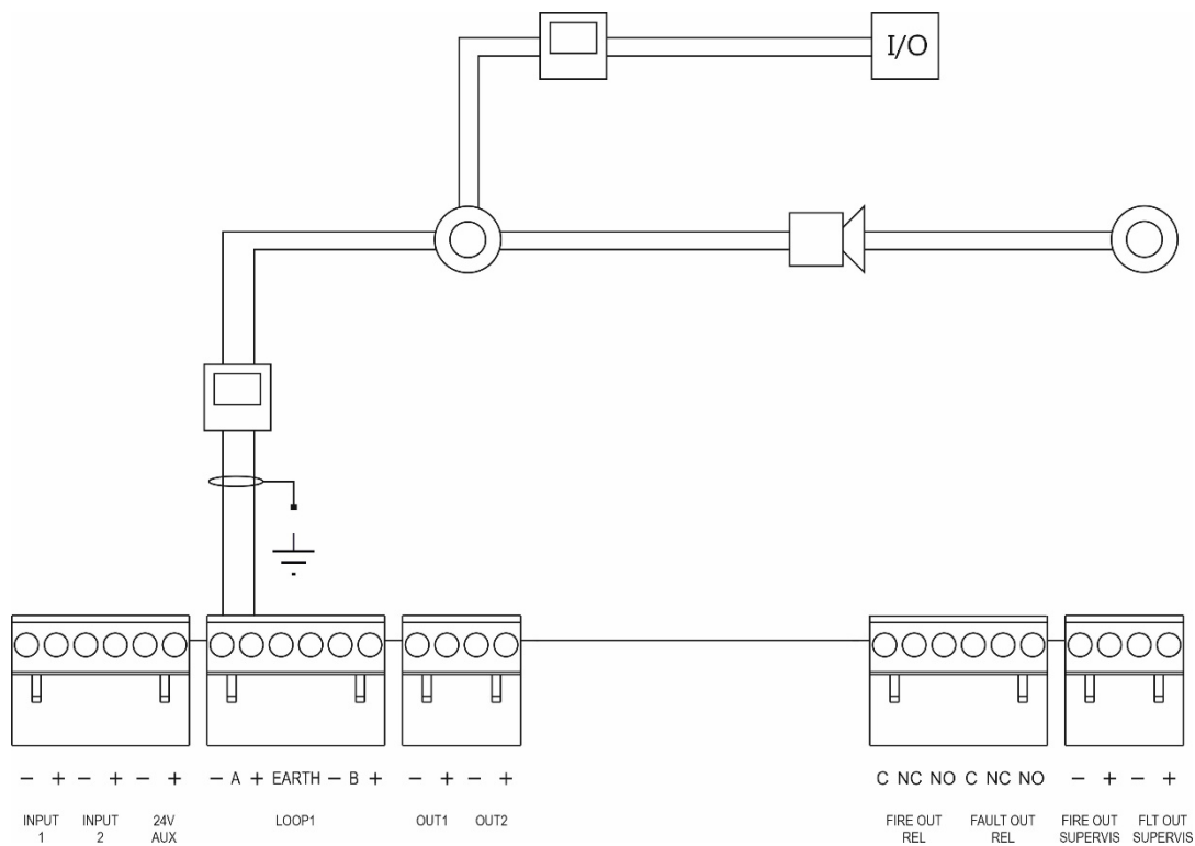
Figura 16: Ligação do loop da Classe B
