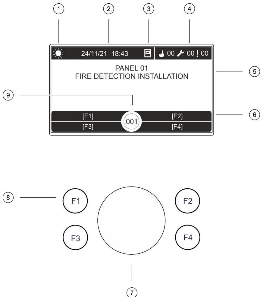
Figura 3: Controlos e indicadores do LCD
