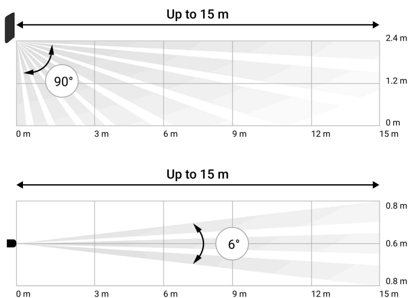
Ângulos de visão horizontal e vertical do detetor
